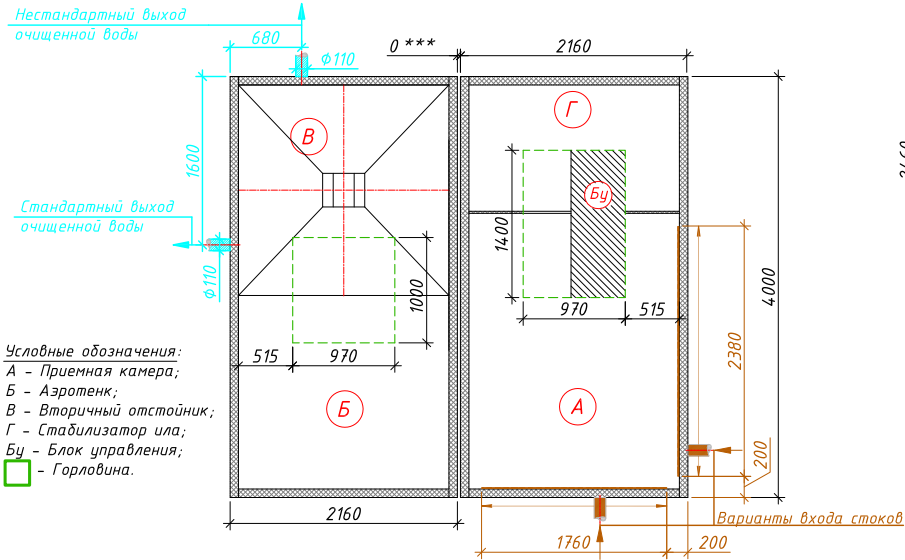
Схема станции
